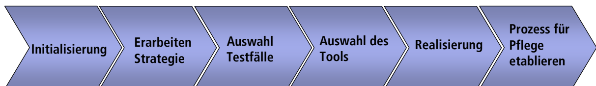
Ablauf Testautomatisierung
