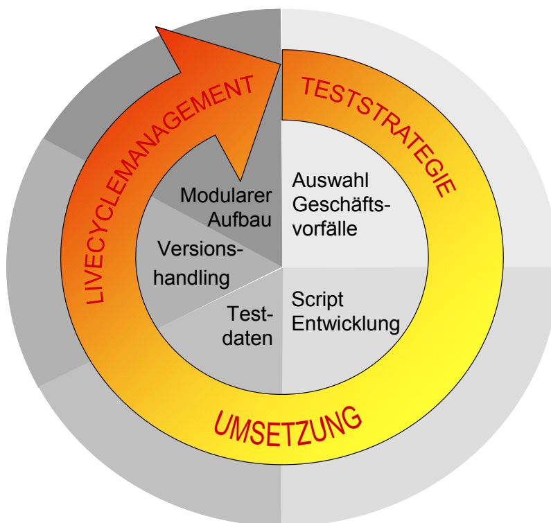
Framework Testautomatisierung
